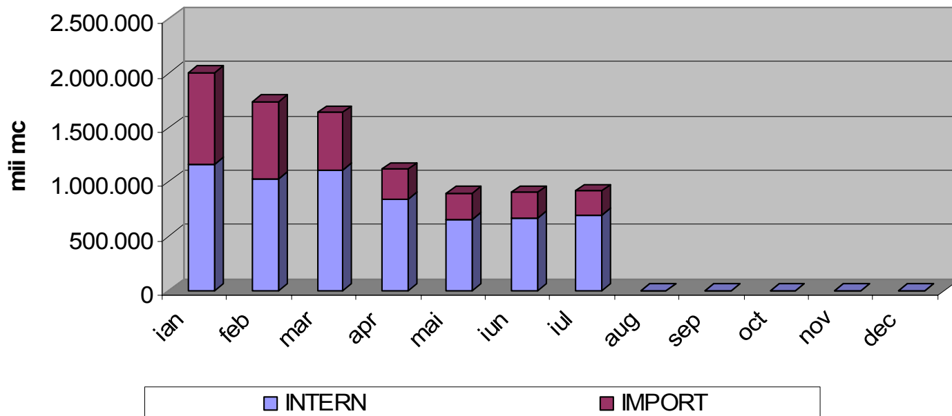
Consumul intern lunar și acoperirea cu gaze naturale (intern, import)
