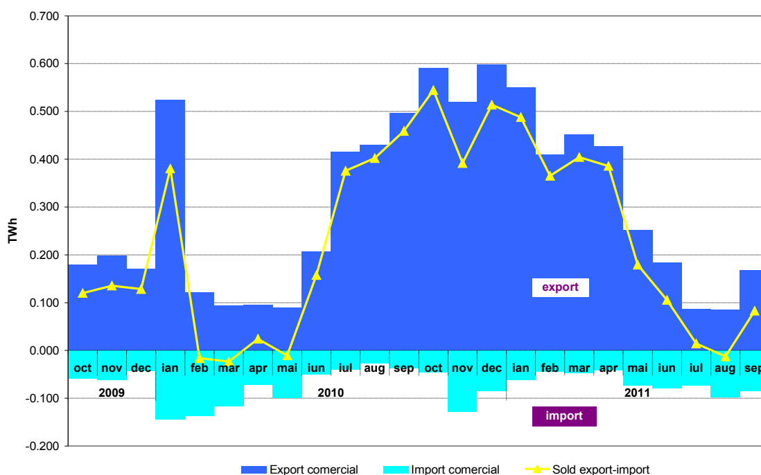
Evolutia lunara a exportului, importului si soldului export-import de energie electrica in ultimele 24 luni
