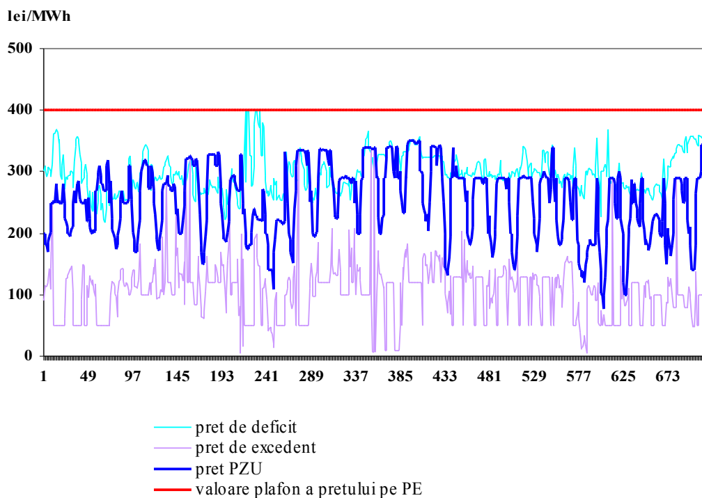
Preturi orare de decontare luna Septembrie 2011
