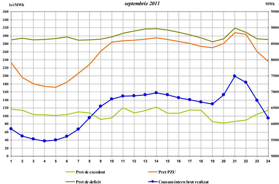
Valori medii orare ale preturilor de decontare si ale consumului intern brut realizat septembrie 2011
