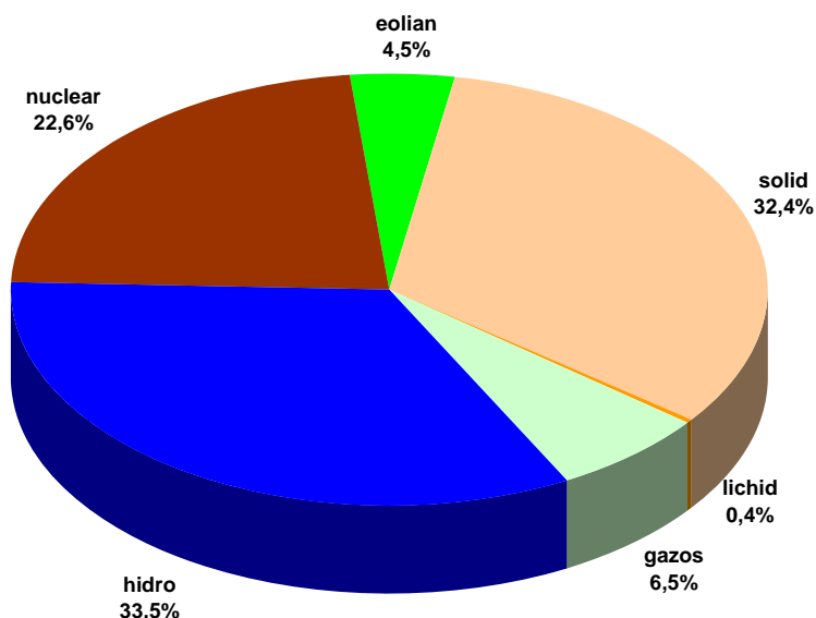
Structura pe tipuri de resurse a energiei electrice livrate in rețele de producătorii cu unitati dispecerizabile - aprilie 2012-
