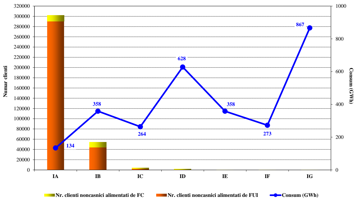
Numărul clienților noncasnici și consumul lor structurat pe tranșe de consum și tip furnizor - MAI 2021 -
