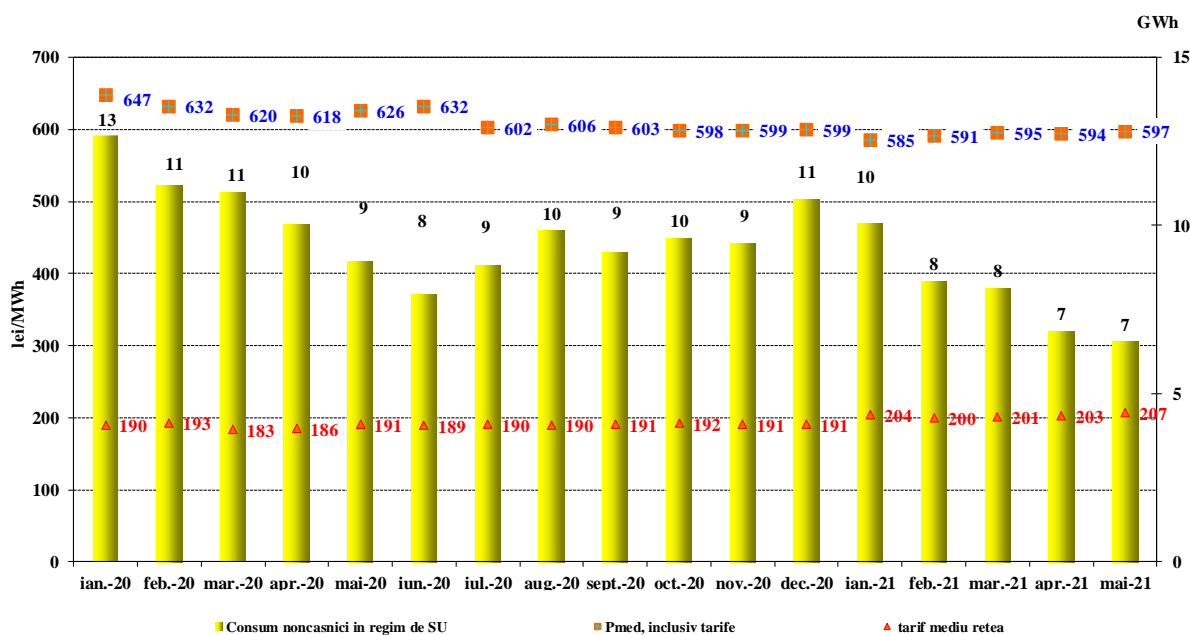
Evoluție lunară a prețului mediu vânzare, a tarifului mediu și a consumului de energie electrică pentru clienții noncasnici alimentați în regim SU - Ianuarie 2020 - Mai 2021 -
