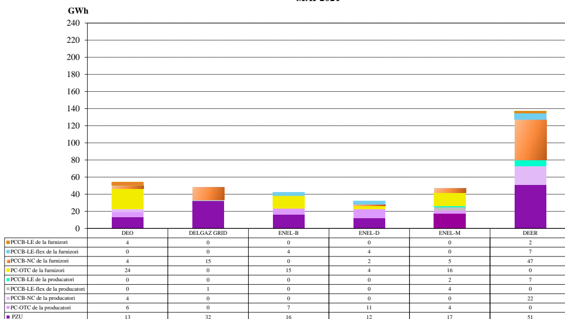
Structura achizițiilor de energie electrică ale operatorilor de distribuție concesionari pentru acoperirea consumului propriu tehnologic - MAI 2021 -
