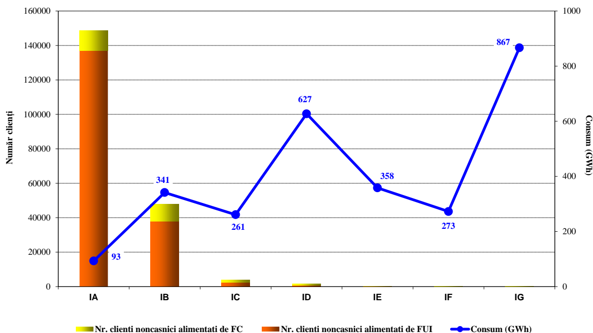
Numărul clienților noncasnici alimentați în regim concurențial și consumul lor structurat pe tranșe de consum și tip furnizor - MAI 2021 -
