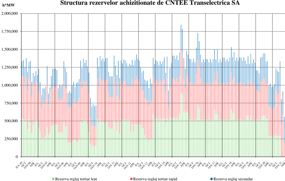
Structura rezervelor achiziționate de CNTEE Transelectrica SA
