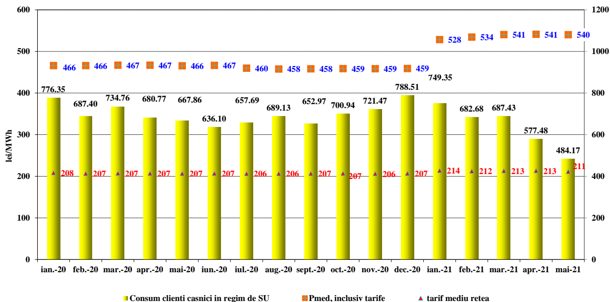
Evoluție lunară a prețului mediu de vânzare și a consumului de energie electrică pentru clienții casnici - Ianuarie 2020 - Mai 2021 -
