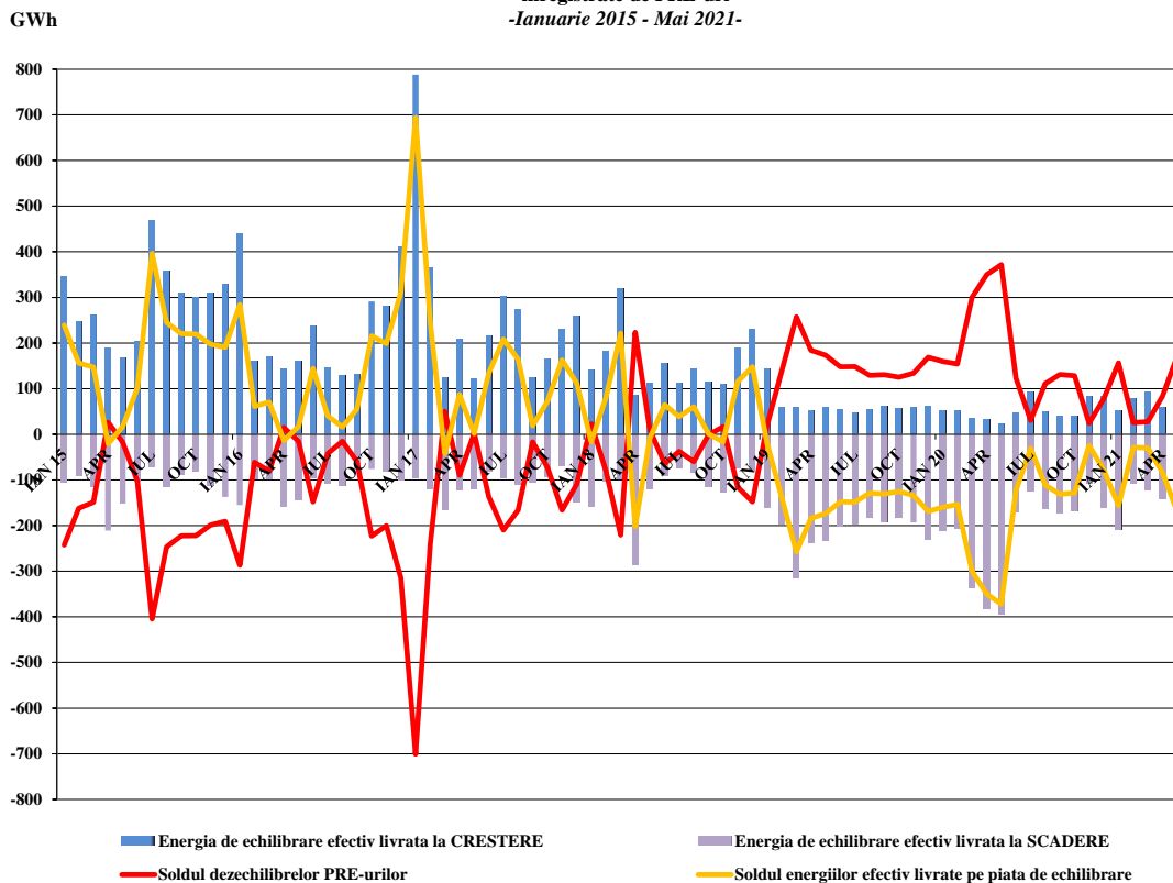
Evoluția lunară a energiei de echilibrare efectiv livrată și a soldului rezultat comparativ cu soldul dezechilibrului înregistrate de PRE-uri -Ianuarie 2015 - Mai 2021-
