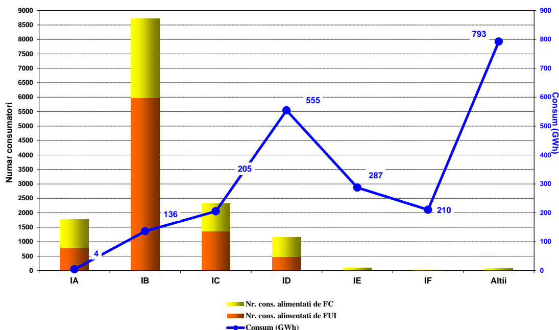
Numarul consumatorilor alimentati in regim concurential si consumul lor structurat pe categorii de consum si furnizori - IULIE 2013 -
