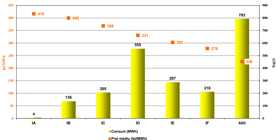
Pretul mediu si consumul de energie structurat pe categorii de consumatori corespunzator segmentului concurential al PAM IULIE 2013 -
