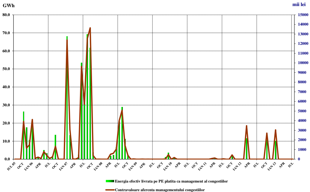
Evoluția lunară a energiei efectiv livrata pe piața de echilibrare pentru managementul congestiilor pe liniile interne și a contravalorii acesteia
