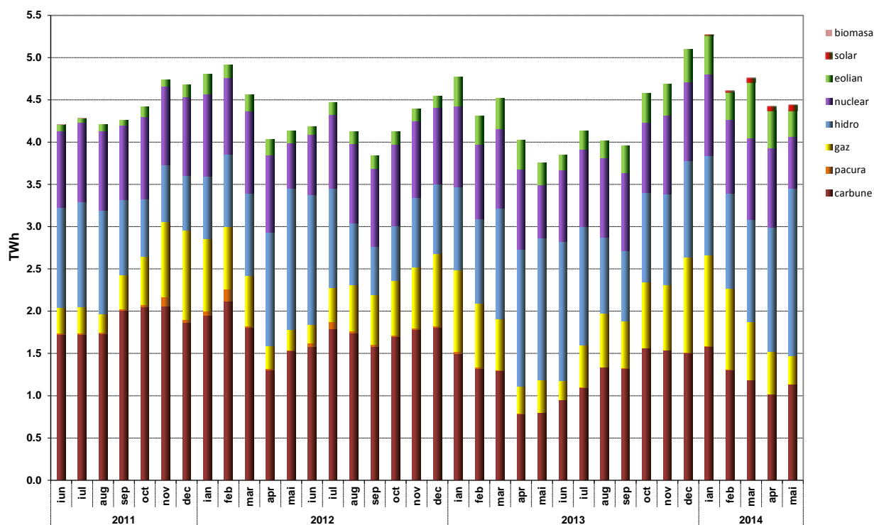
Evoluția structurii pe tipuri de resurse a energiei electrice livrate în rețea de producătorii cu unități dispatchabile
