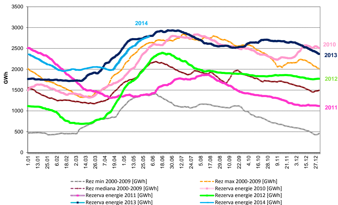
Evoluția comparativă pe durata unui an a rezervei de energie zilnică în principalele lacuri de acumulare
