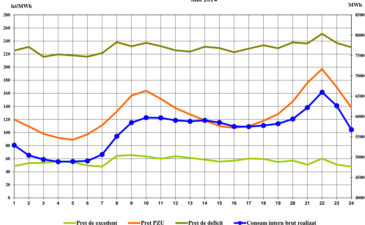
Valori medii orare ale preturilor de decontare și ale consumului intern brut realizat Mai 2014
