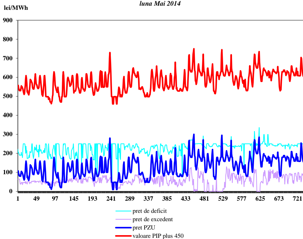
Preturi orare de decontare luna Mai 2014
