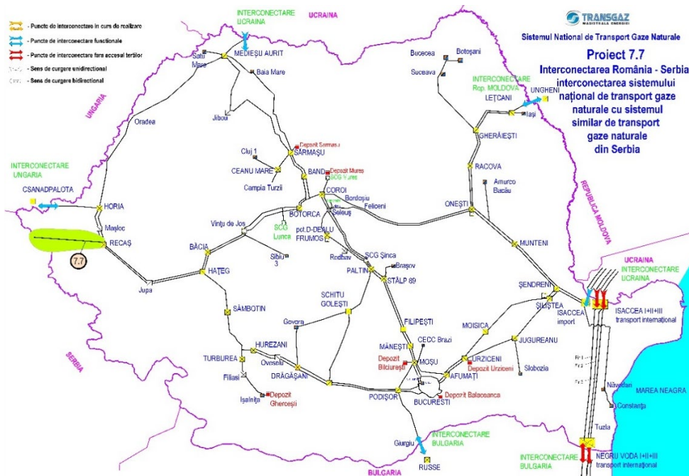
Figura 14 - Interconectarea SNT cu Serbia pe direcția Recaș–Mokrin
