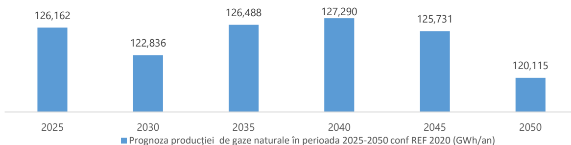
Grafic 12 – Prognostul producției de gaze naturale în perioada 2025-2050 conform Scenariului de referință al Comisiei Europene(REF 2020)
