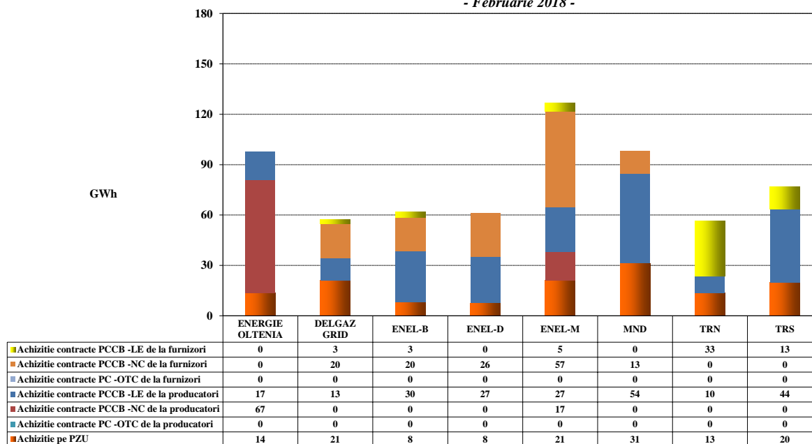
Structura tranzacțiilor de energie electrică ale operatorilor de distribuție principali corespunzătoare acoperirii consumului propriu tehnologic - Februarie 2018 -
