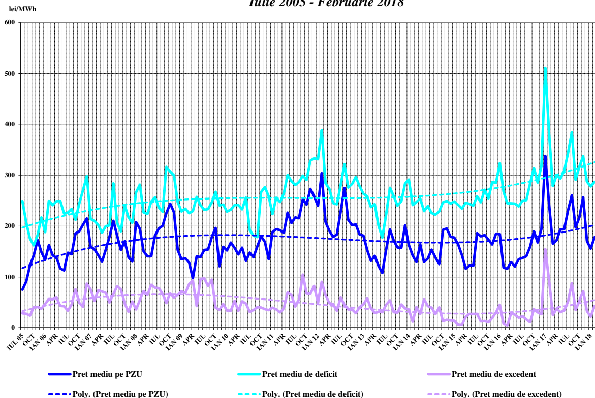
Preturi medii lunare inregistrate pe PZU si PE Iulie 2005 - Februarie 2018
