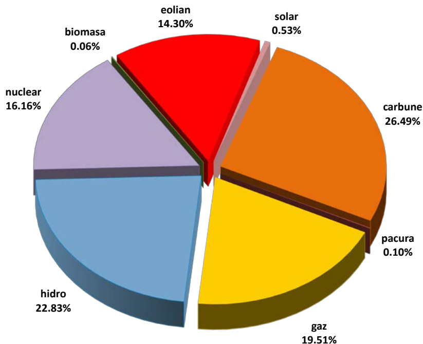
Structura pe tipuri de resurse a energiei electrice livrate în rețele de producătorii cu unitati dispecerizabile - Februarie 2018 -
