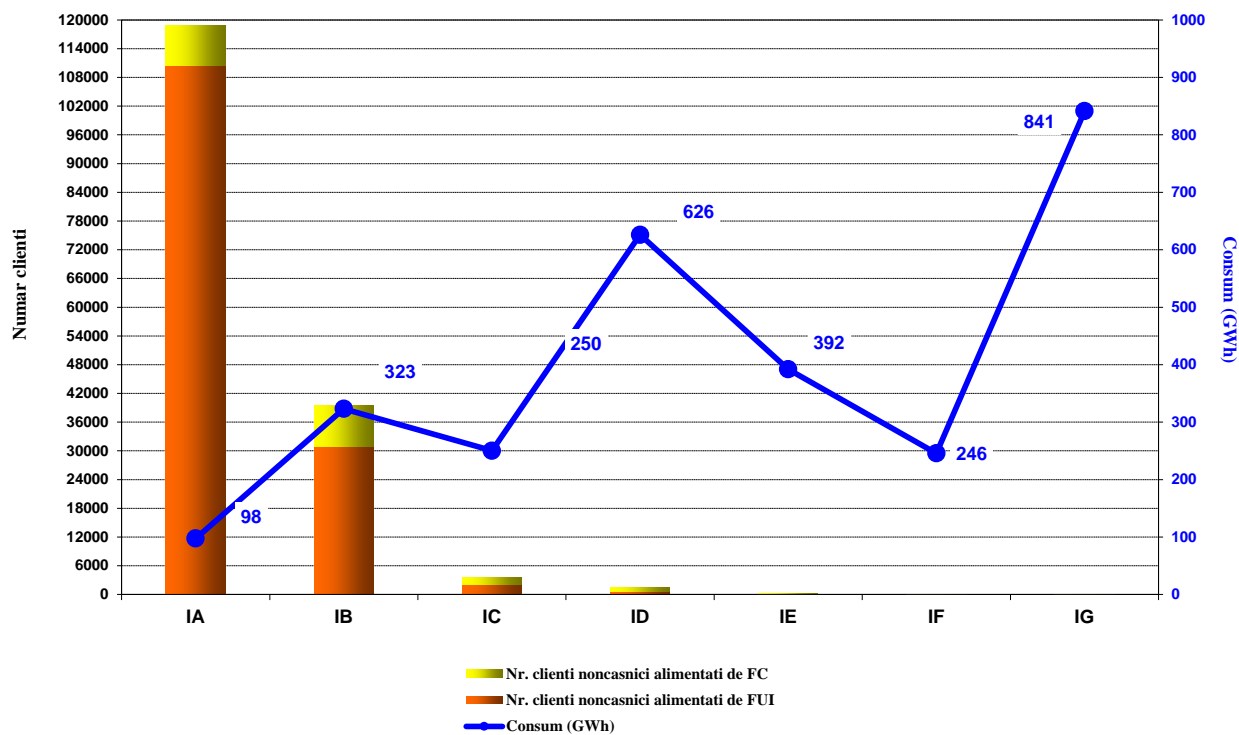
Numărul clienților noncasnici alimentați în regim concurențial și consumul lor structurat pe tranșe de consum și tip furnizor - APRILIE 2018 -
