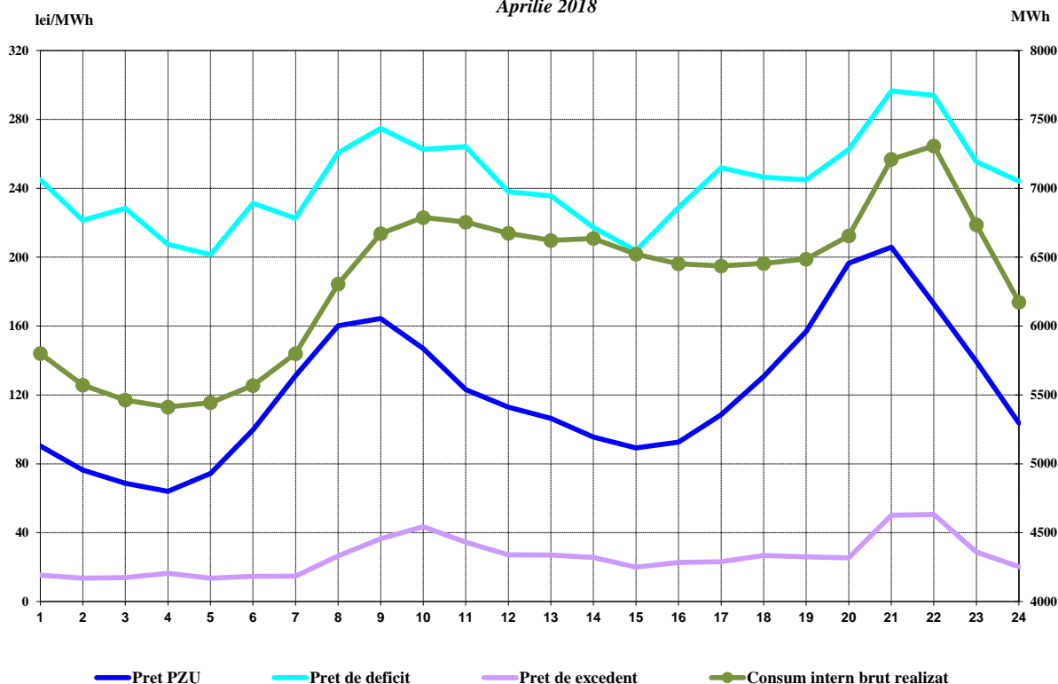
Valori medii orare ale preturilor de decontare si ale consumului intern brut realizat Aprilie 2018
