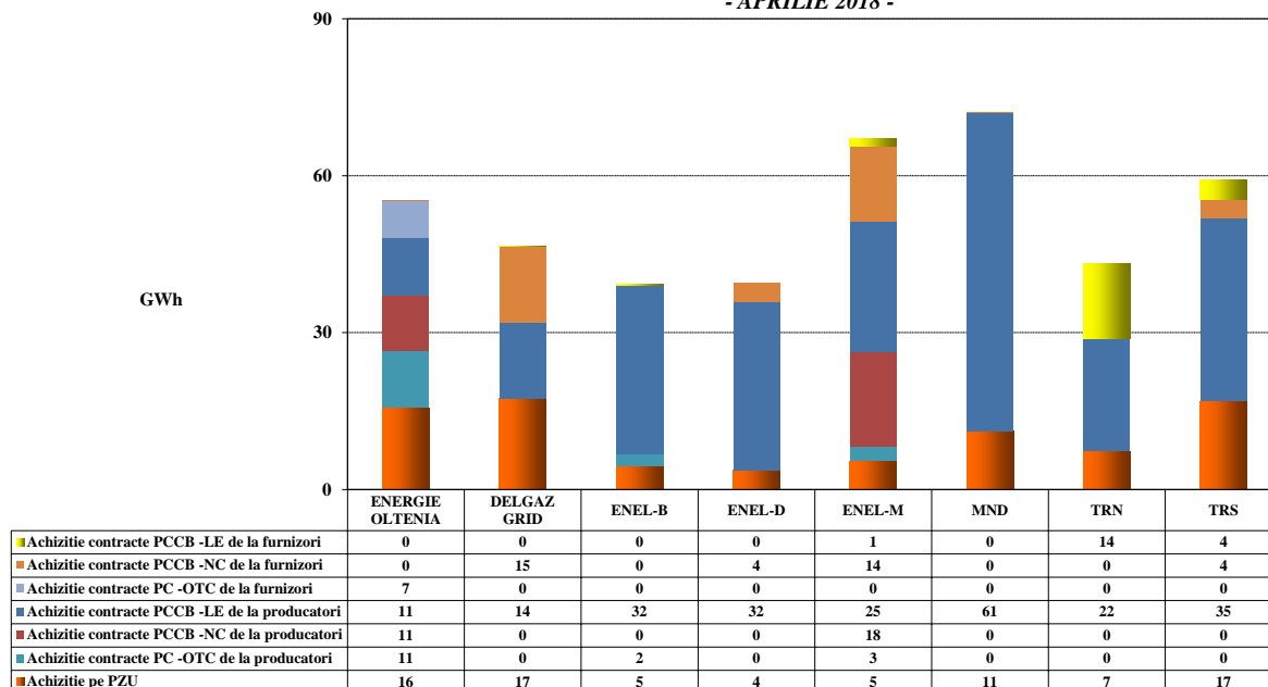
Structura tranzacțiilor de energie electrică ale operatorilor de distribuție principali corespunzătoare acoperirii consumului propriu tehnologic - APRILIE 2018 -
