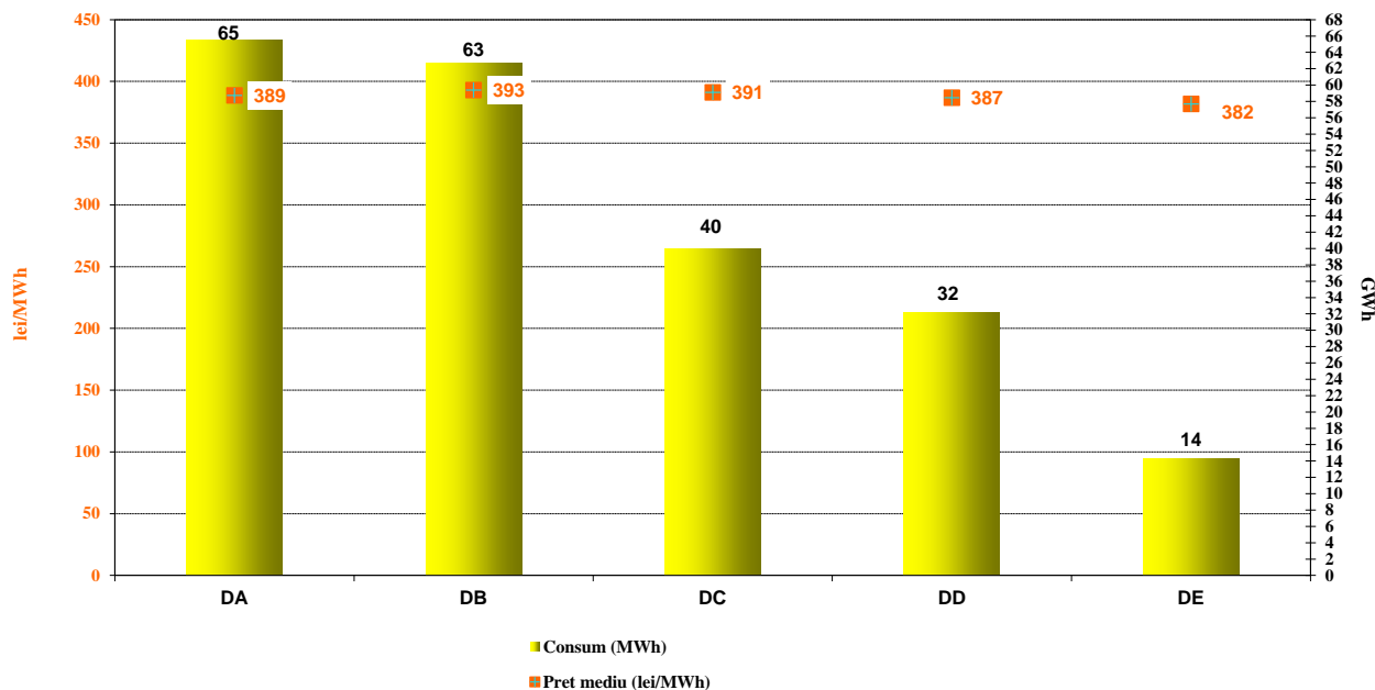
Prețul mediu și consumul de energie electrică structurat pe tranșe de consum pentru clienții casnici pe segmentul concurențial al PAM - APRILIE 2018 -
