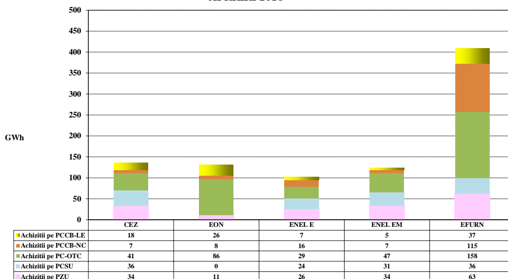
Structura tranzacțiilor furnizorilor de ultimă instanță pentru clienții finali alimentați în regim SU și UI - APRILIE 2018-
